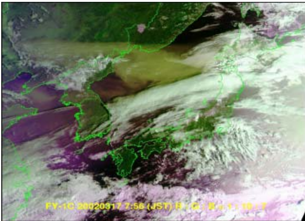
図7 FY-1C画像(2002年3月17日受信:黄色部分は大陸から 黄砂が朝鮮半島や日本海へ飛来する様子を示す)
