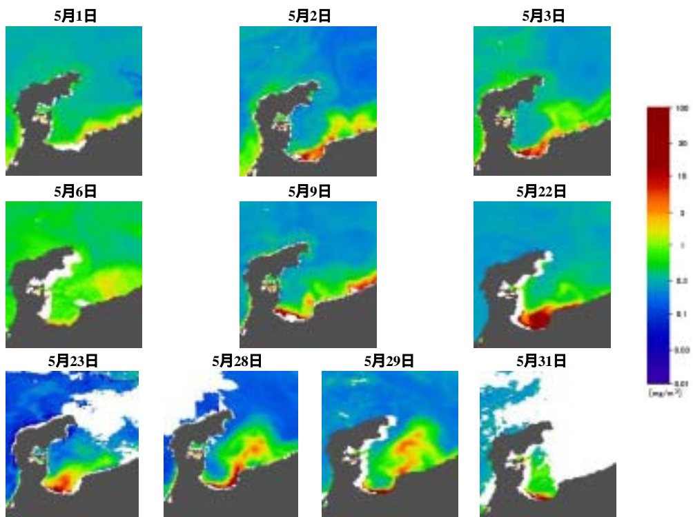
図3 MODISの水色データを活用した富山湾のクロロフィルa濃度の時系列変動(2003年)
