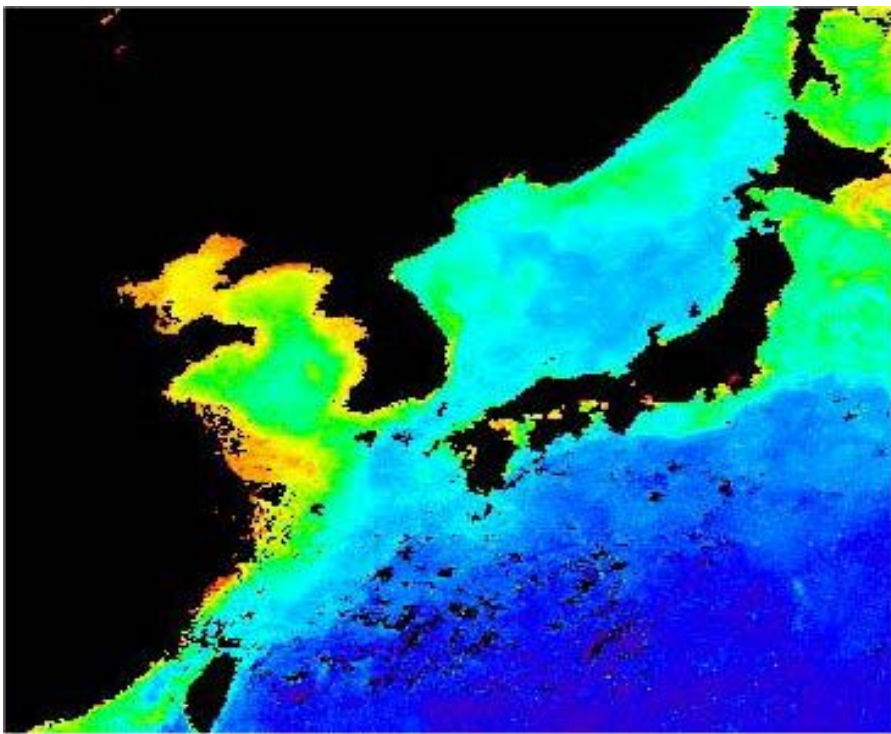
図5 日本海・黄海海域のクロロフィルa濃度(2002年6月)
